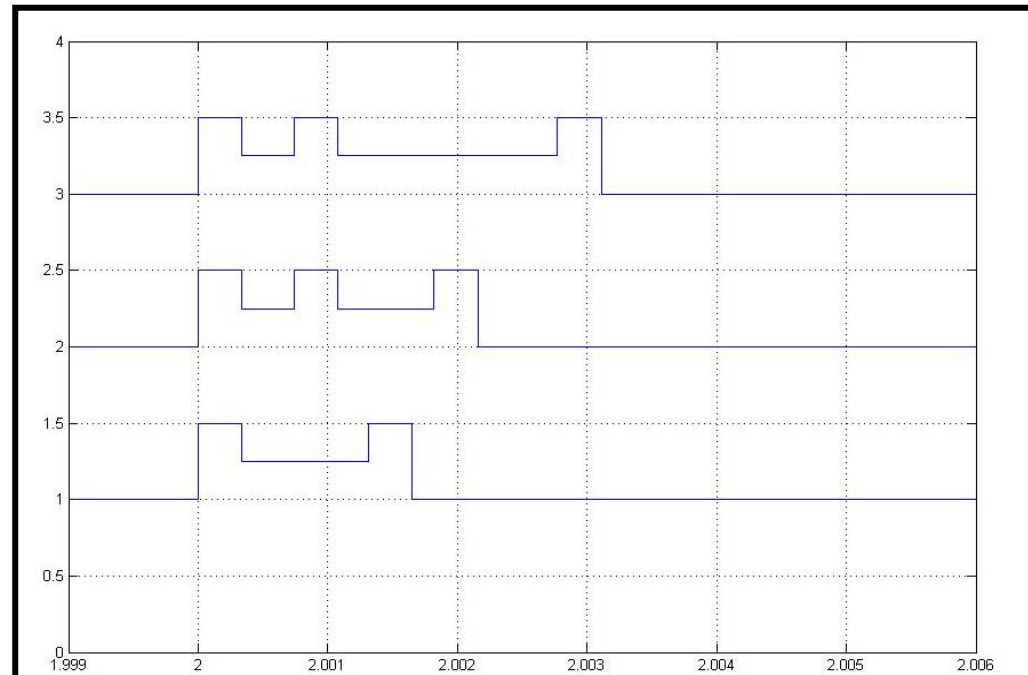
Vremenski dijagrami slanja pojedinih čvorova
